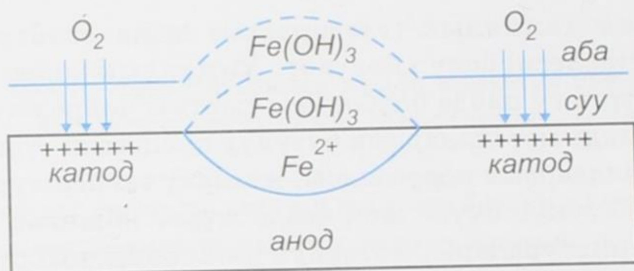
7.5-сурет. Темир коррозиясынын схемасы.
