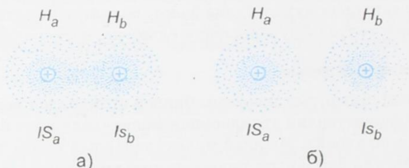
3.4-сүрөт. Коваленттик молекуладагы булуттун жайгашуу схемасы.
